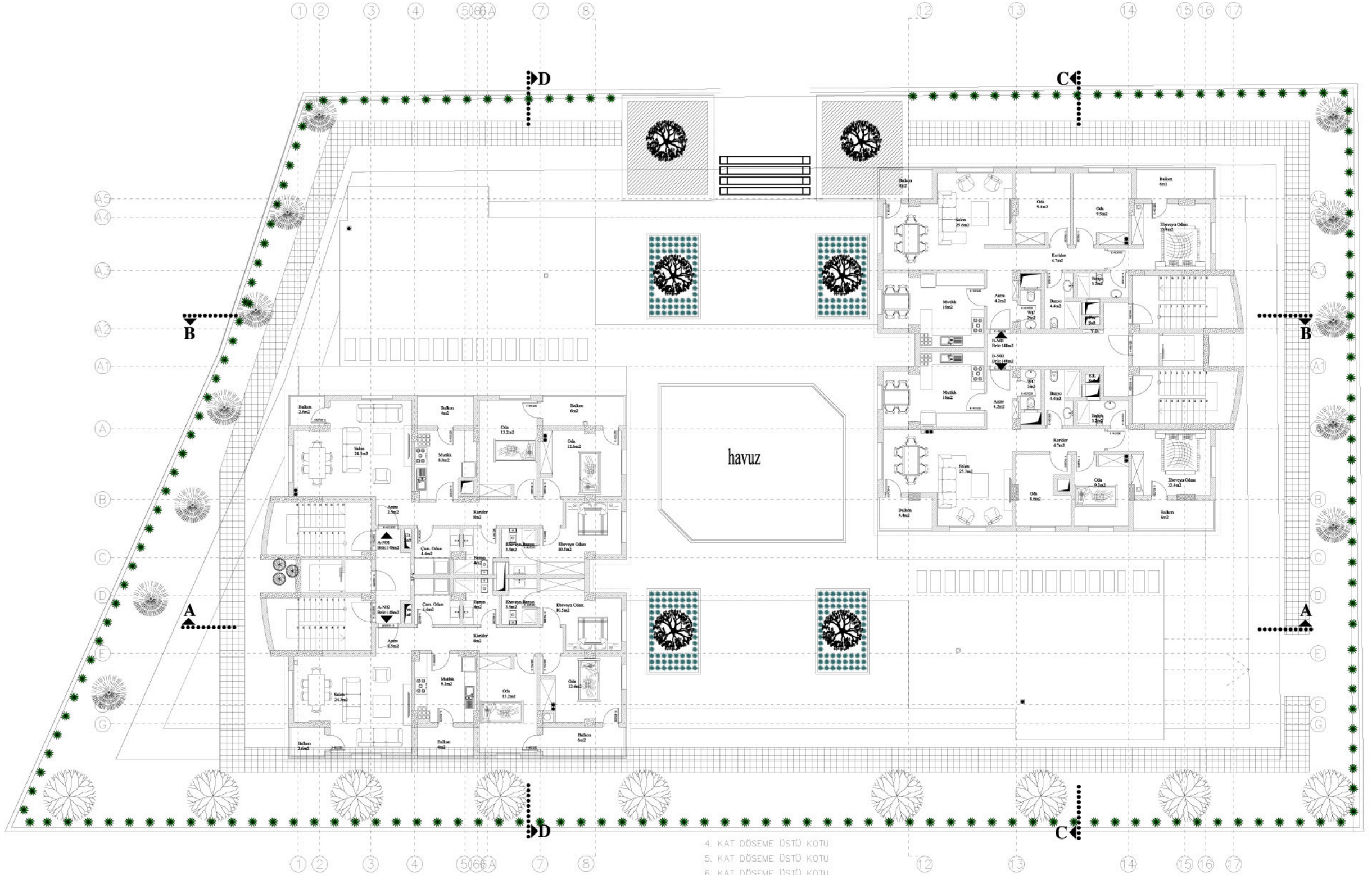
(4-5-6-7-8-9) NORMAL KAT PLANI Ölçek 1/50
